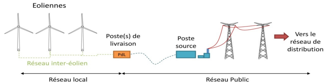
Figure 1 : Raccordement électrique des installations (Source : Guide de l'étude de dangers des parcs éoliens, Juin 2012)
